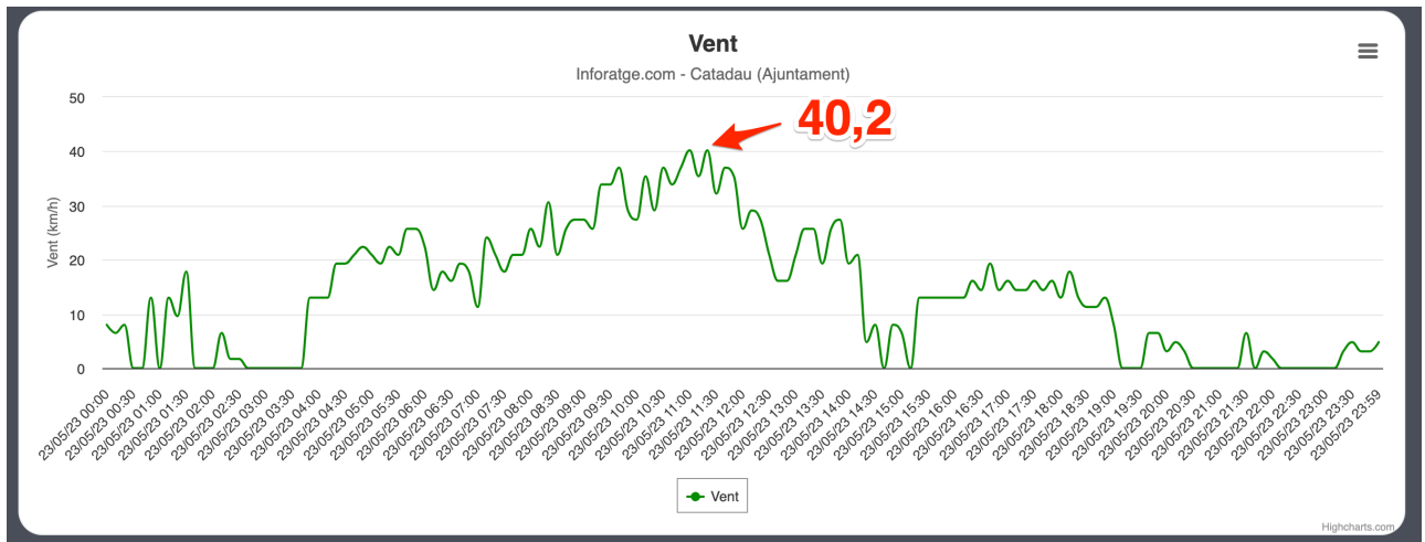
Ráfagas de viento registradas en CATADAU (estación "núcleo urbano") el 23/05/23 (en km/h) https://inforatge.com/meteo-catadau
