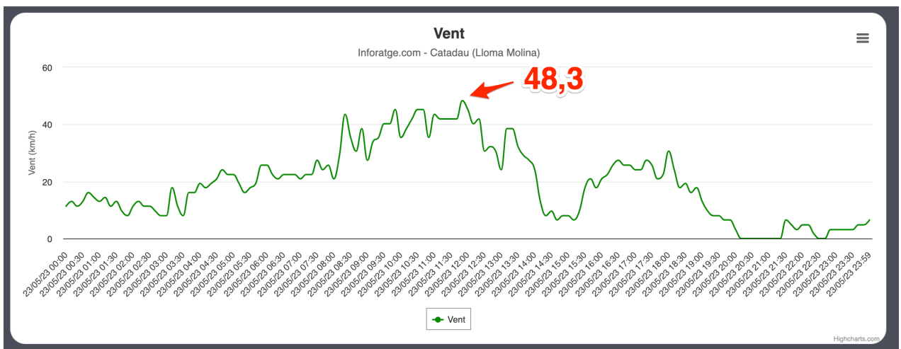
Ráfagas de viento registradas en CATADAU (estación "Lloma Molina") el 23/05/23 (en km/h) https://inforatge.com/meteo-catadau
