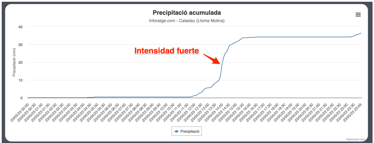
Evolución lluvia acumulada en CATADAU (Loma Molina) el 23/05/23 (en l/m 2 ) https://inforatge.com/meteo-catadau
