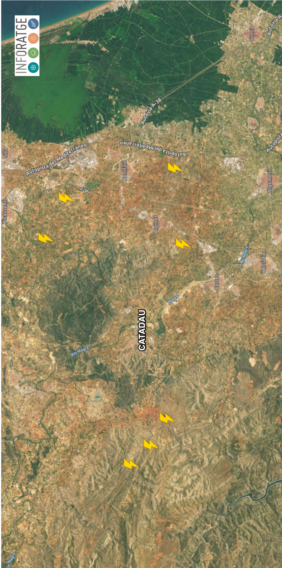
Geolocalización de las descargas eléctricas ` nube-tierra` registradas en el término municipal de CATADAU y alrededores el 23/05/23 Fuente descargas: www.lightningmaps.org // Cartografía: © Instituto Geográfico Nacional de España
